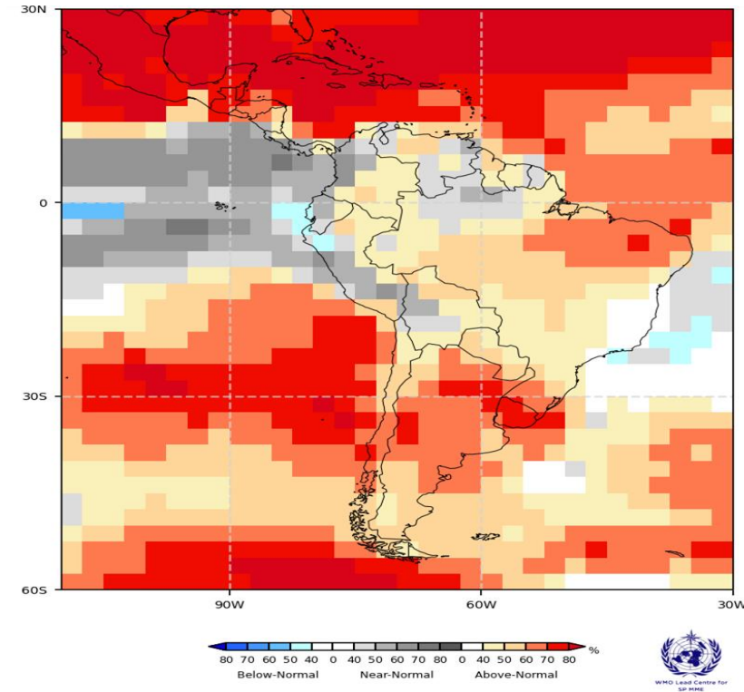
Figura 07 – Previsão probabilística da temperatura (DJF)
