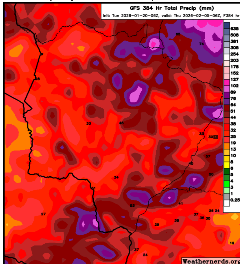
Figura 08 - Precipitação acumulada prevista do modelo GFS
