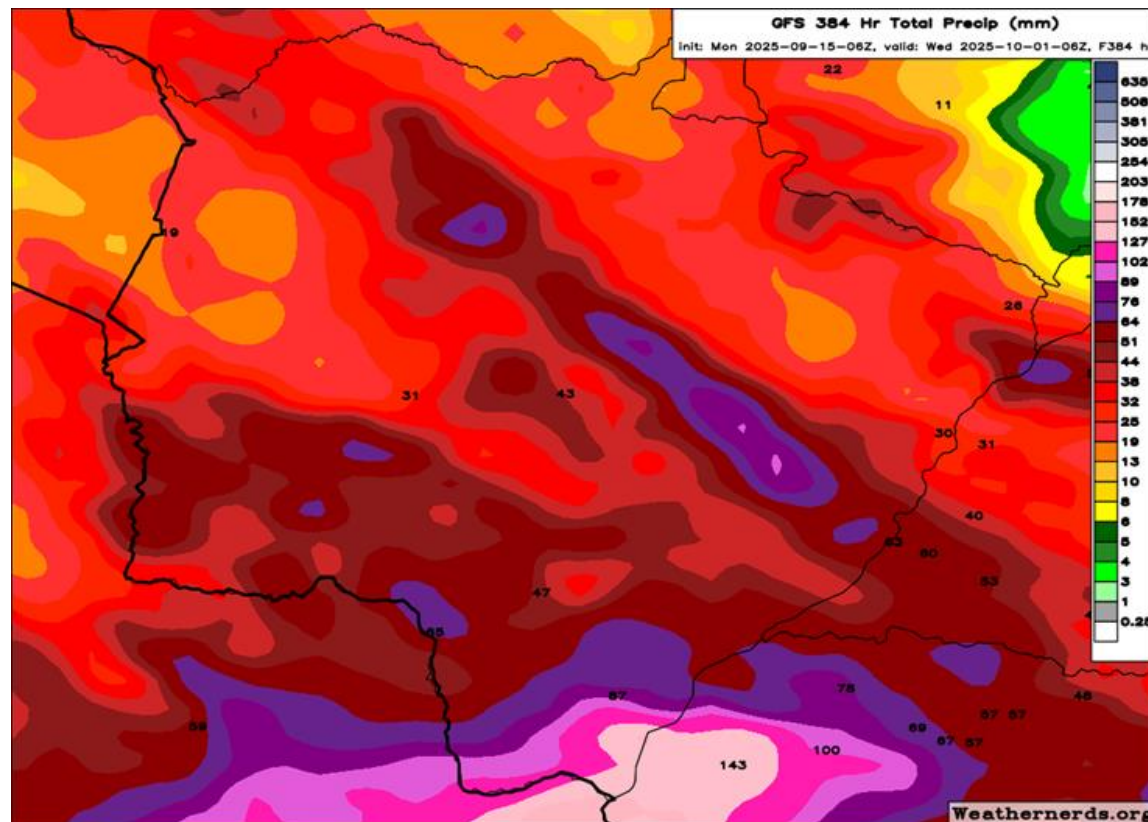
Figura 10 - Precipitação acumulada prevista do modelo GFS
