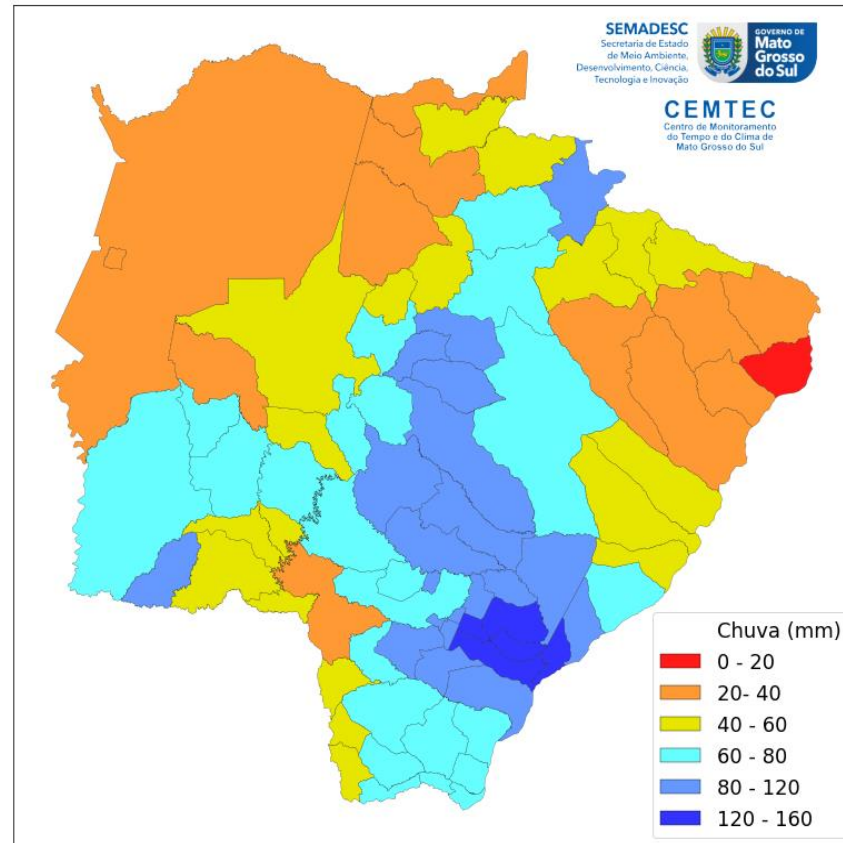
Figura 02 – Precipitação acumulada
