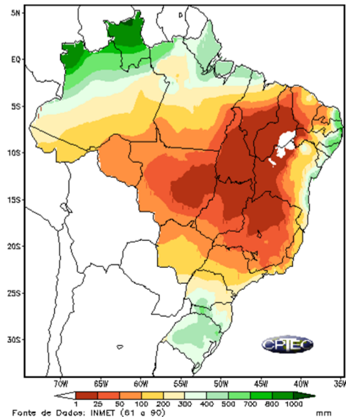
Figura 06 – Média climatológica (JJA)
