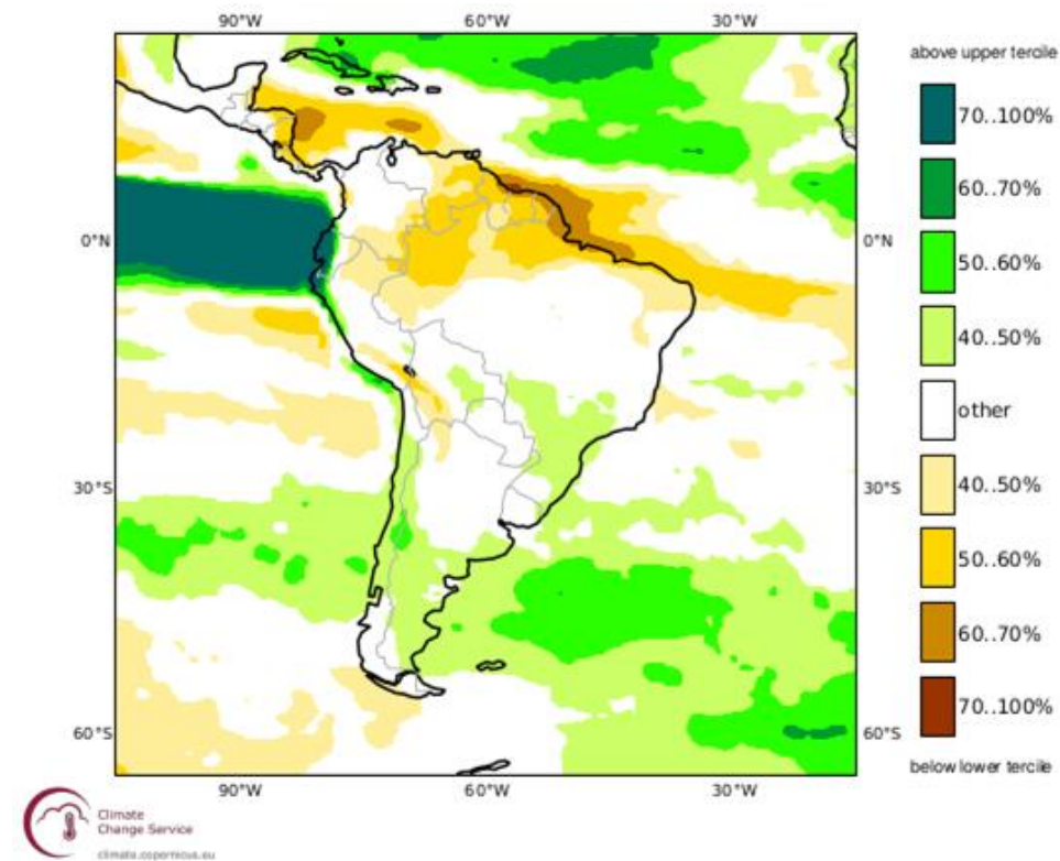
Figura 07 – Previsão probabilística (JJA)
