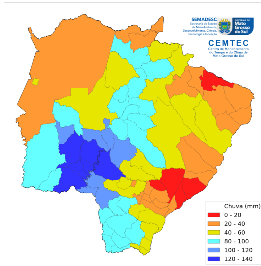
Figura 02 – Precipitação acumulada
